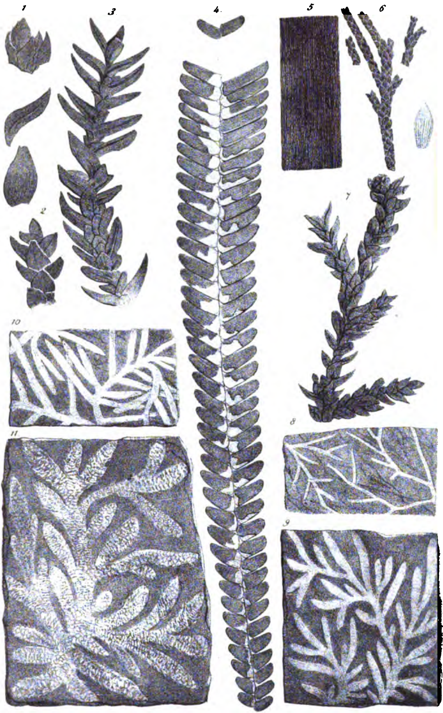
Quenstedt, Jura.
